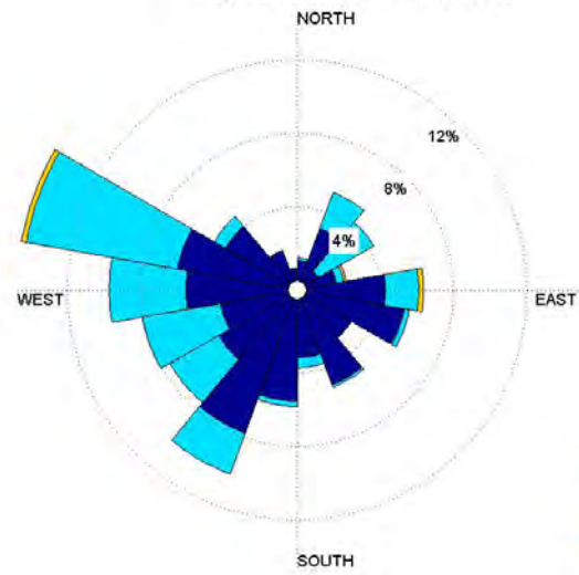
Byvind, Yttre Hanöbukten april 2010
