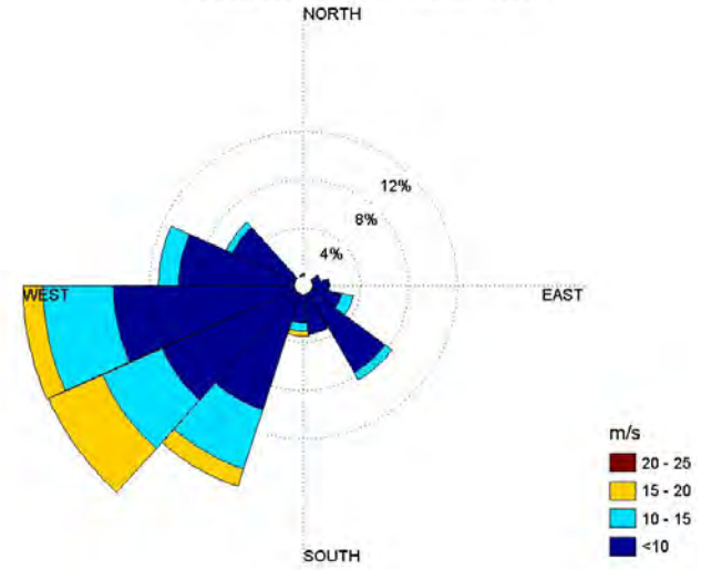
Byvind, Inre Hanöbukten september 2011
