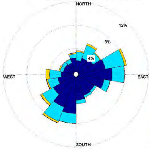
Byvind, Vindstationen Hanø april 1999-2009
