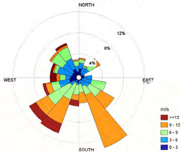
Medelvind, Yttre Hanöbukten oktober 2010
