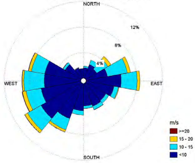
Byvind, Yttre Hanöbukten maj 1999-2009
