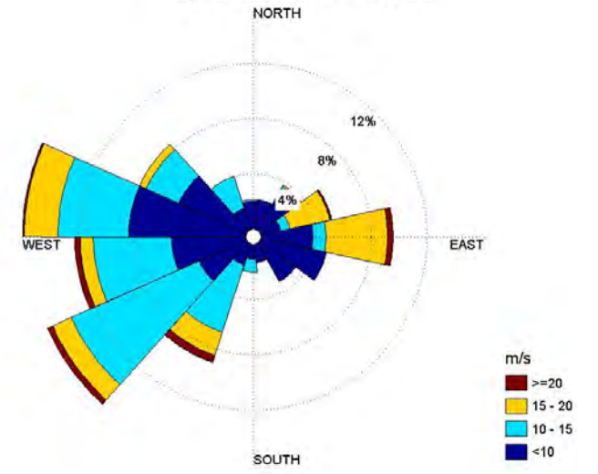
Byvind, Yttre Hanöbukten mars 2011
