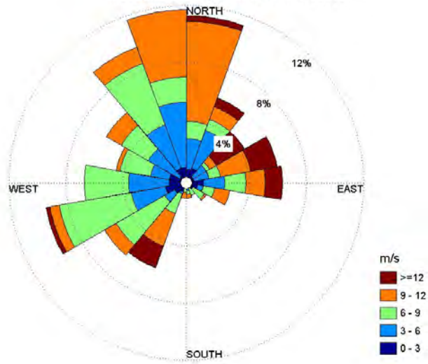
Medelvind, Inre Hanöbukten december 2010
