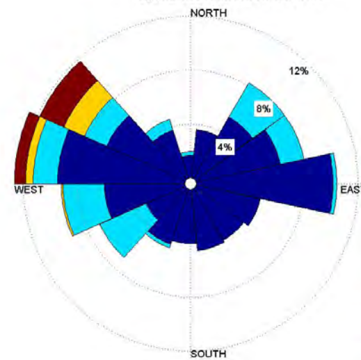
Byvind, Inre Hanöbukten april 2011
