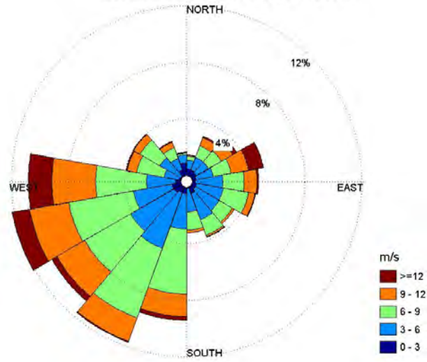
Medelvind, Vindstationen Hanö juni 1999-2009
