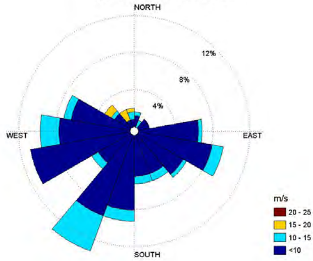
Byvind, Vindstationen Hanö juli 2010
