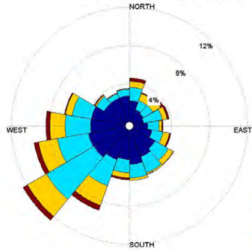
Byvind, Yttre Hanöbukten oktober 1999-2009
