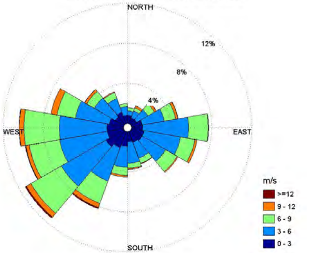
Medelvind, Inre Hanöbukten augusti 1999-2009
