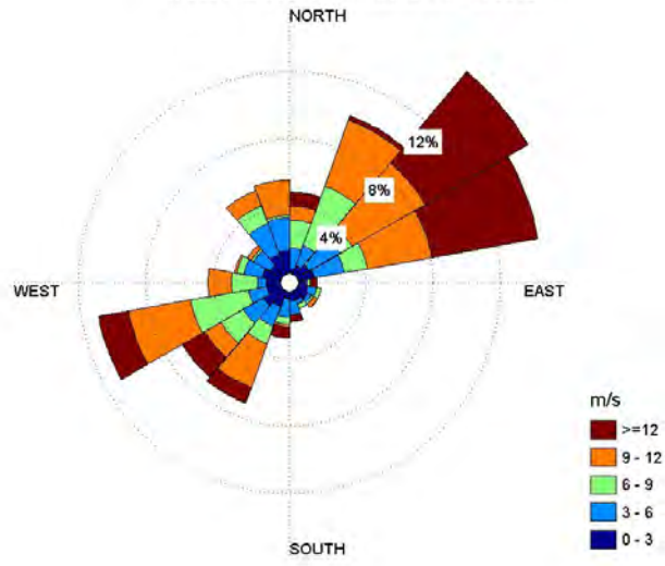
Medelvind, Inre Hanöbukten november 2010
