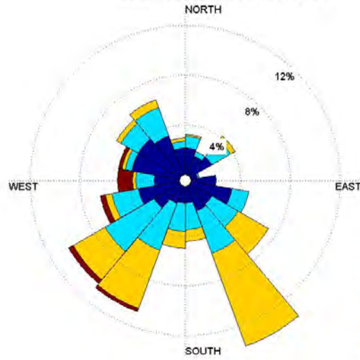
Byvind, Yttre Hanöbukten oktober 2010
