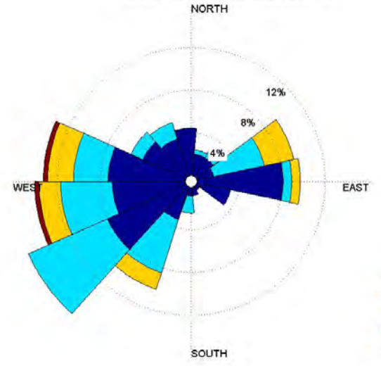
Byvind, Vindstationen Hanø mars 2011
