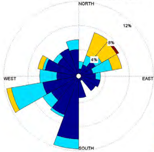
Byvind, Vindstationen Hanö maj 2010
