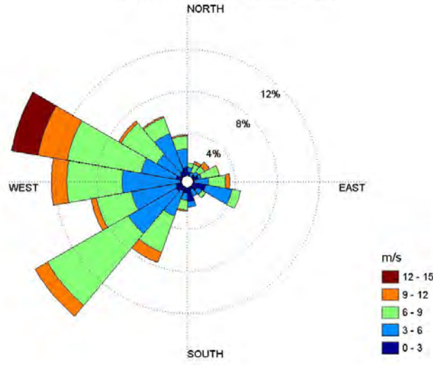
Medelvind, Yttre Hanöbukten mars 2010
