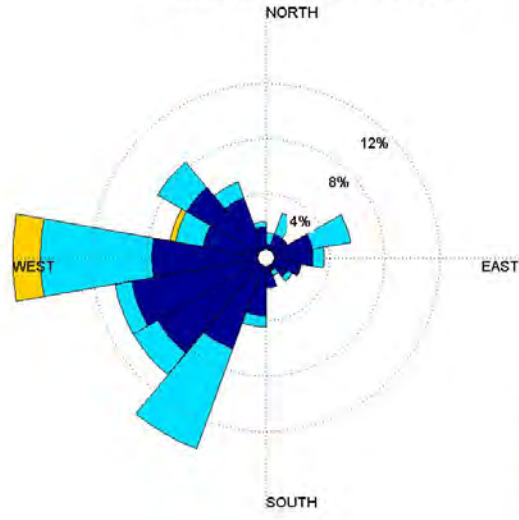
Byvind, Vindstationen Hanø mars 2010
