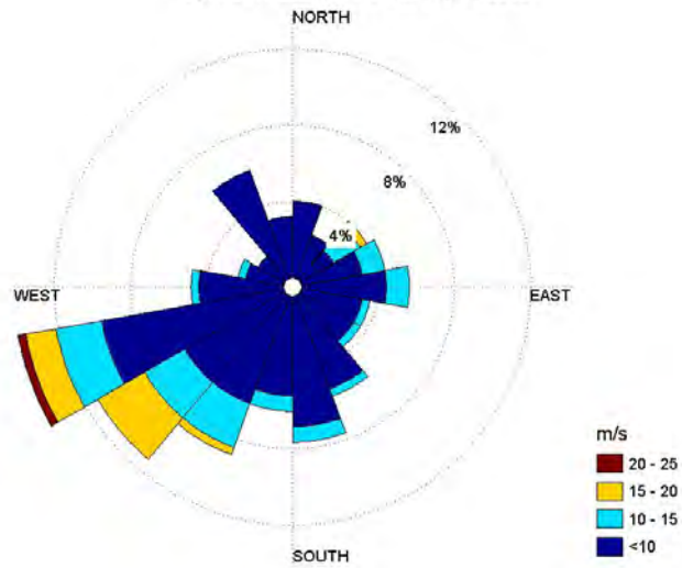
Byvind, Vindstationen Hanö augusti 2010
