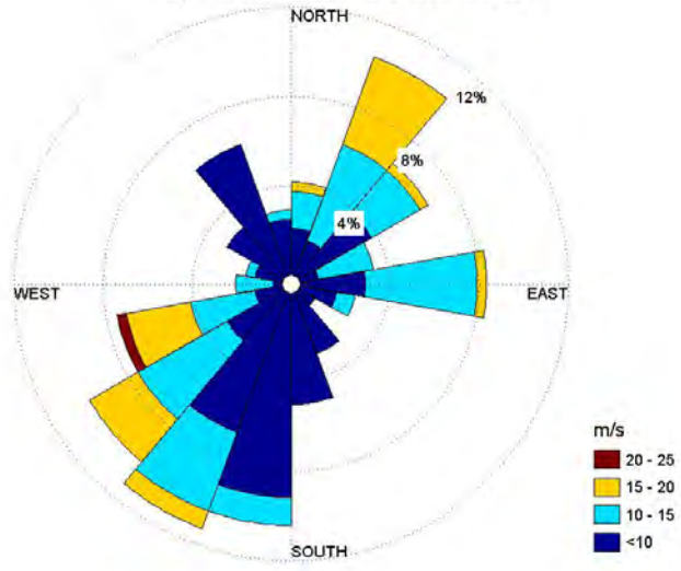
Byvind, Vindstationen Hanó september 2010
