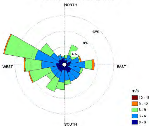
Medelvind, Inre Hanöbukten april 2010
