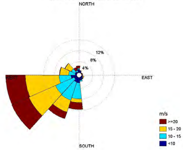
Byvind, Yttre Hanöbukten december 2011
